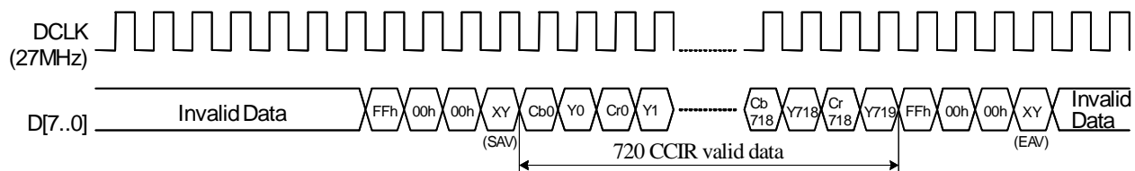
CCIR656 Data input format
